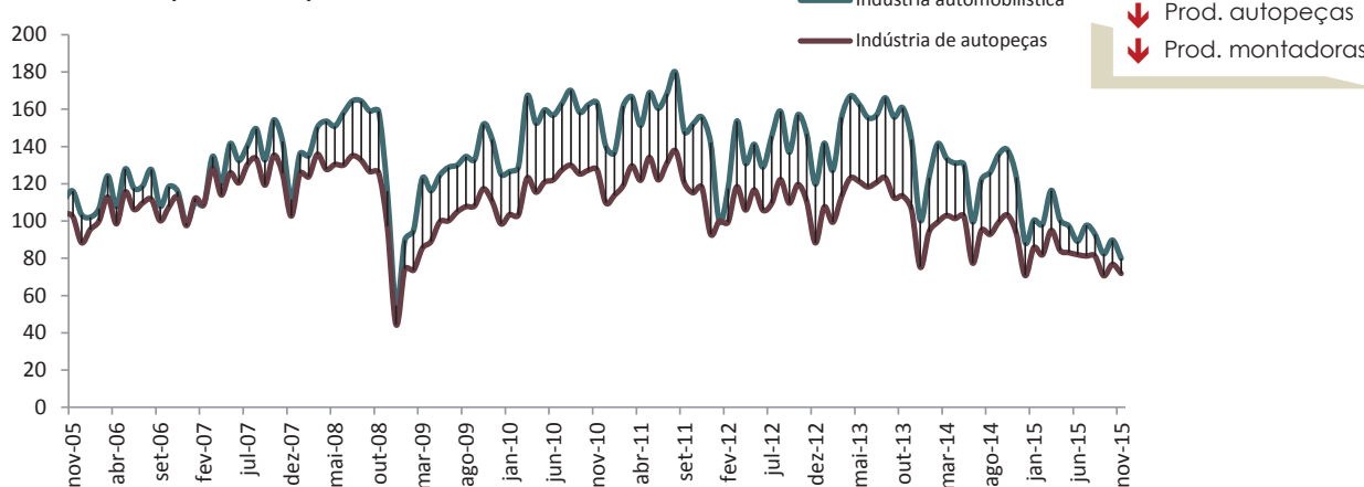
[Gráfico 6] Produção industrial das autopeças x das montadoras Sendo 2012 = 100 (número-índice)
